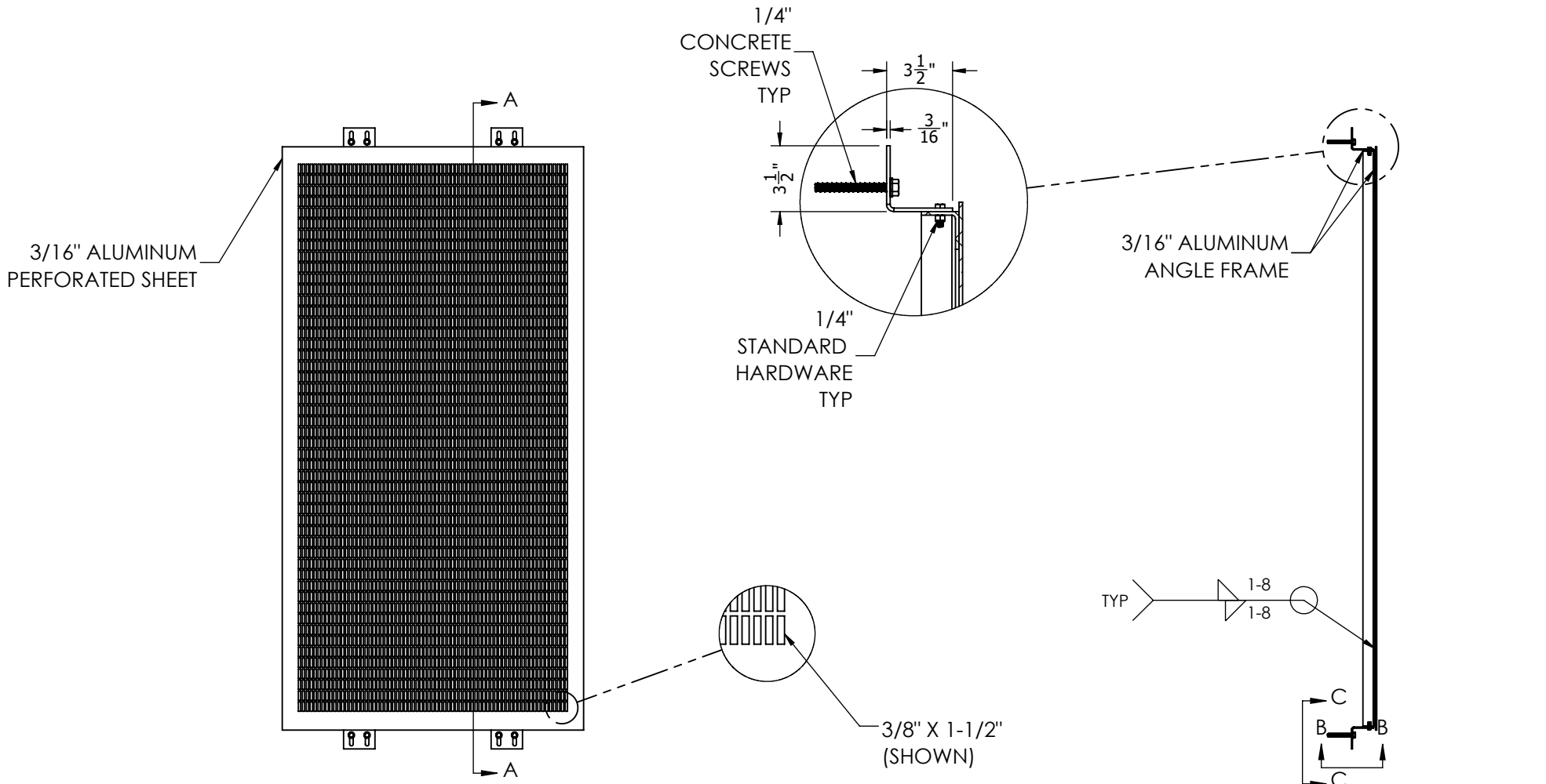
SECTION A-A
